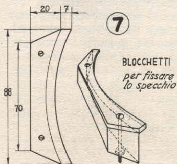
7 Blocchetti ferma specchio.
