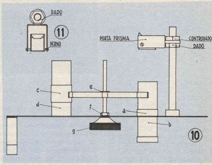
Fig. 10): PIASTRA PORTA-OCULARE, vista di lato. Si osservi il sistema della messa a fuoco. Girando la manopola, e quindi la vite, si determina lo scorrimento del tubo porta-oculare. I tubi a, d, servono da guida affinché lo scorrimento avvenga regolarmente. - Fig. 11): PORTA PRISMA, visio frontalmente. Occorre tenere presente che la parete di questo disti dalla faccia inclinata (ipotenusa) del prisma, almeno 5 mm.
