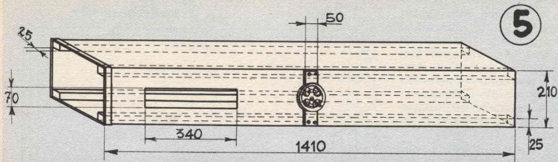
5 Visione d'insieme del tubo dal lato destro. Si notino l'apertura rettangolare e la ruota dentata, fissata ad una fascia, per il movimento verticale
