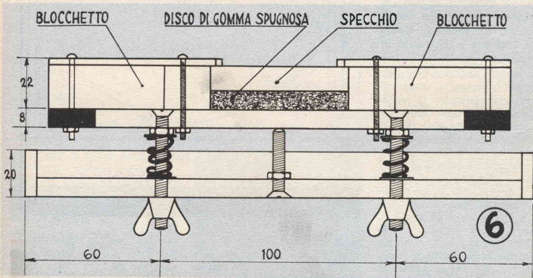
6 SCATOLA PORTA-SPECCHIO, vista come se fosse stata tolta una parete. Sono pure stati messi in evidenza i congegni (viti molle galletti, ecc.) che regolano l'inclinazione dello specchio
