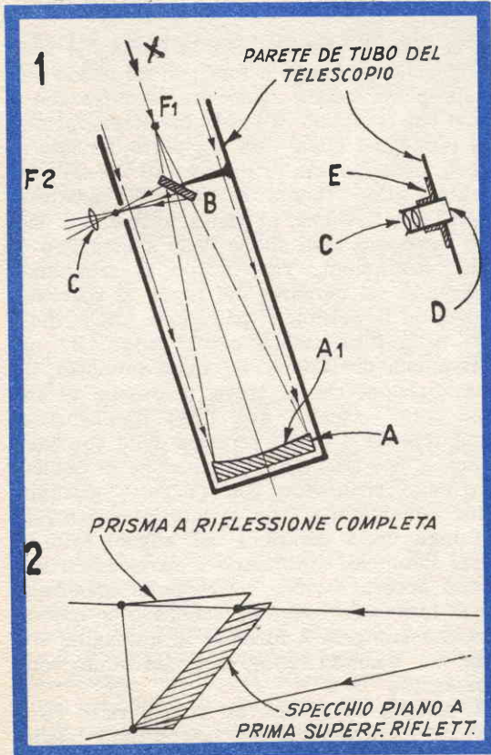
FIG. 1) - Sistema ottico che si attua nel telescopio a riflessione del tipo Newtoniano. FIG. 2) - Comparazione delle caratteristiche di deviazione del cono ottico tra lo specchio piano ed il prisma a riflessione totale.
